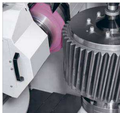
成形研削
